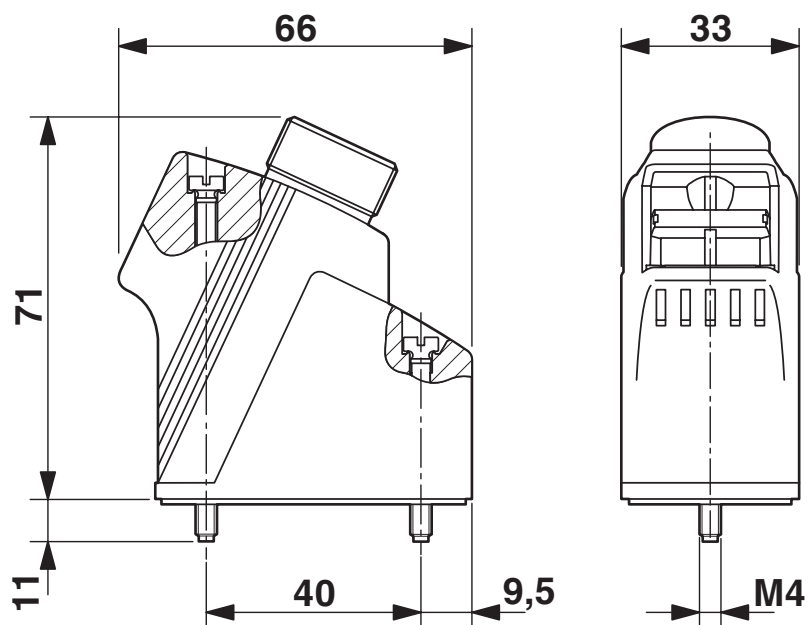
Disegno quotato
