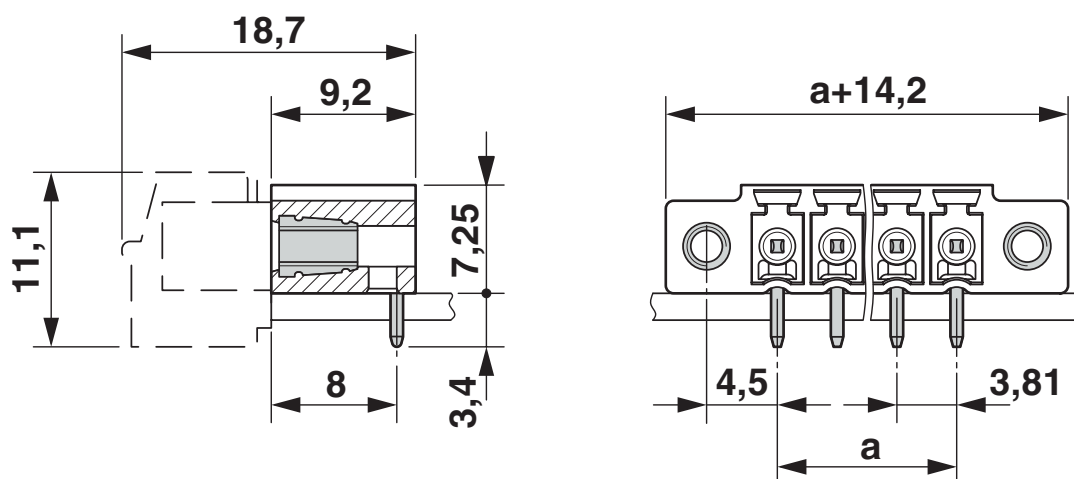
Disegno quotato
