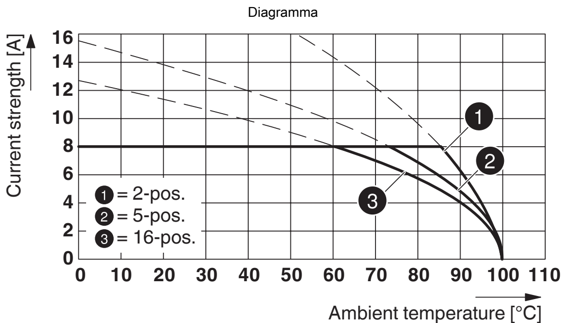
Tipo: FK-MCP 1,5/...-ST-3,81 con MCDV 1,5/...-G1-3,81
