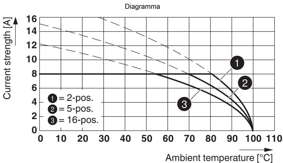
Tipo: FRONT-MC 1,5/...-ST-3,81 con MCDV 1,5/...-G1-3,81
