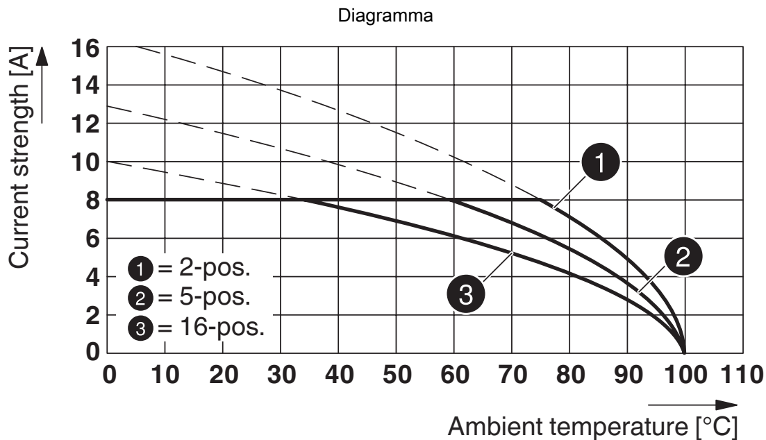
Tipo: MCV(W/R) 1,5/...-ST-3,81 con MCDV 1,5/...-G1-3,81
