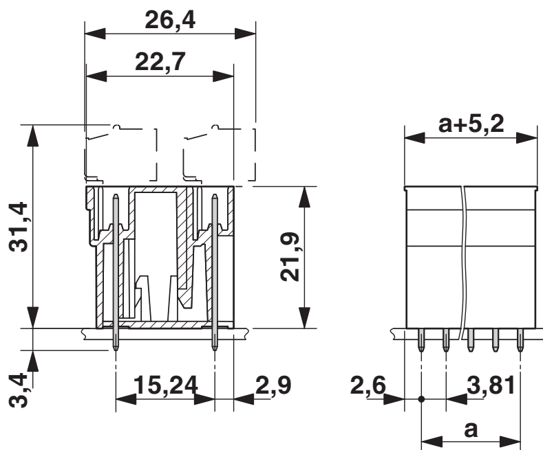
Disegno quotato
