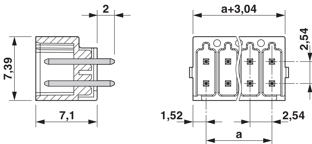
Disegno quotato
