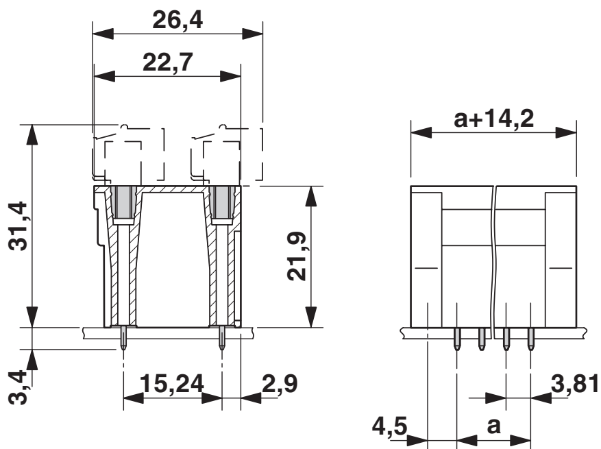
Disegno quotato
