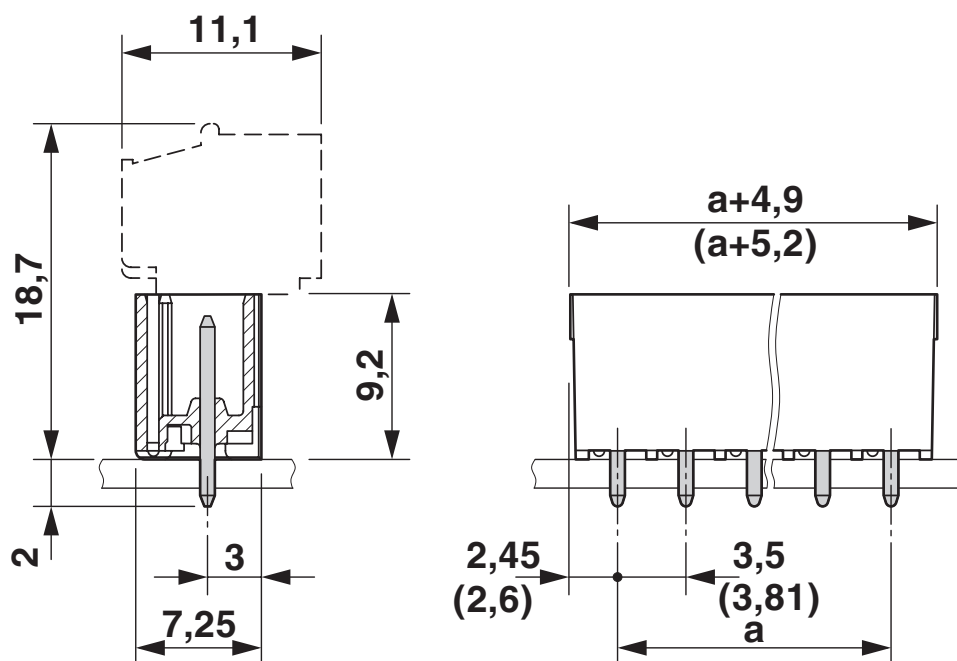
Disegno quotato
