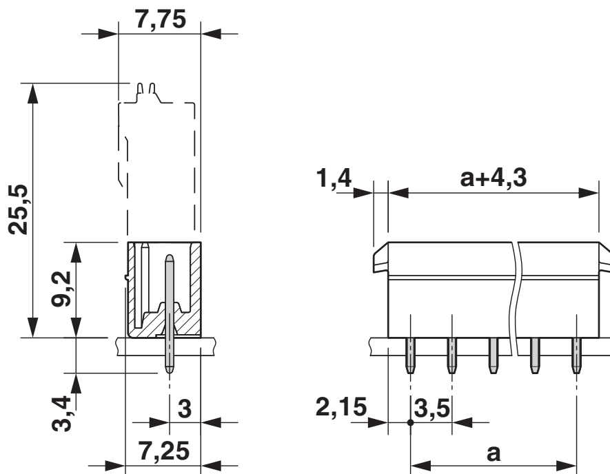
Disegno quotato
