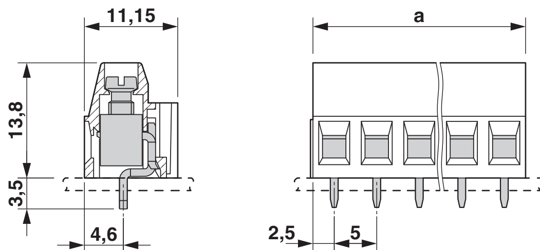
Disegno quotato
