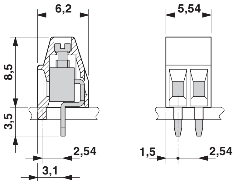
Disegno quotato
