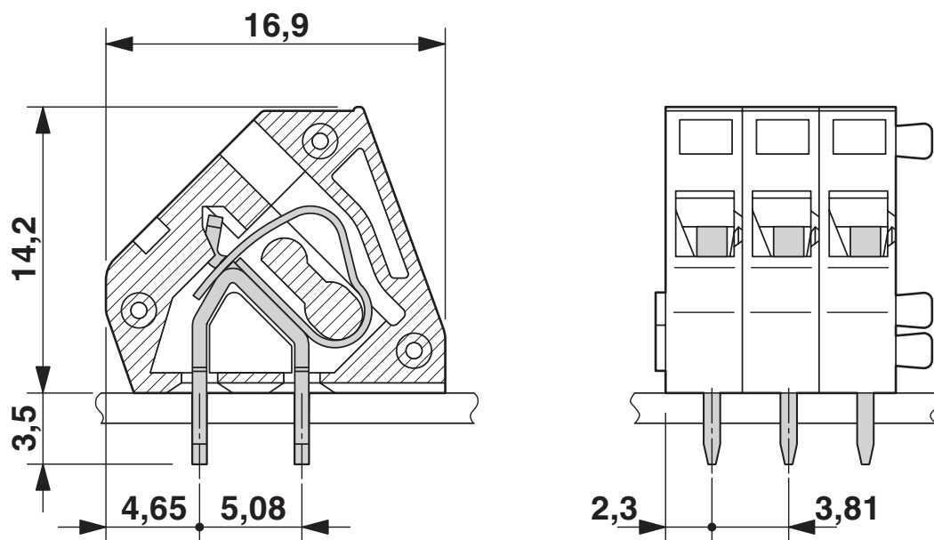
Disegno quotato
