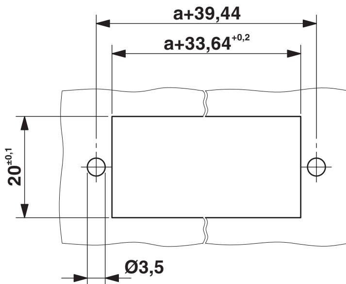
Disegno quotato
