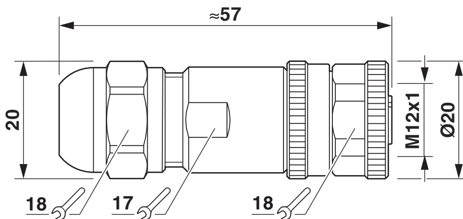
Connettore femmina M12 x 1, diritto, schermato
