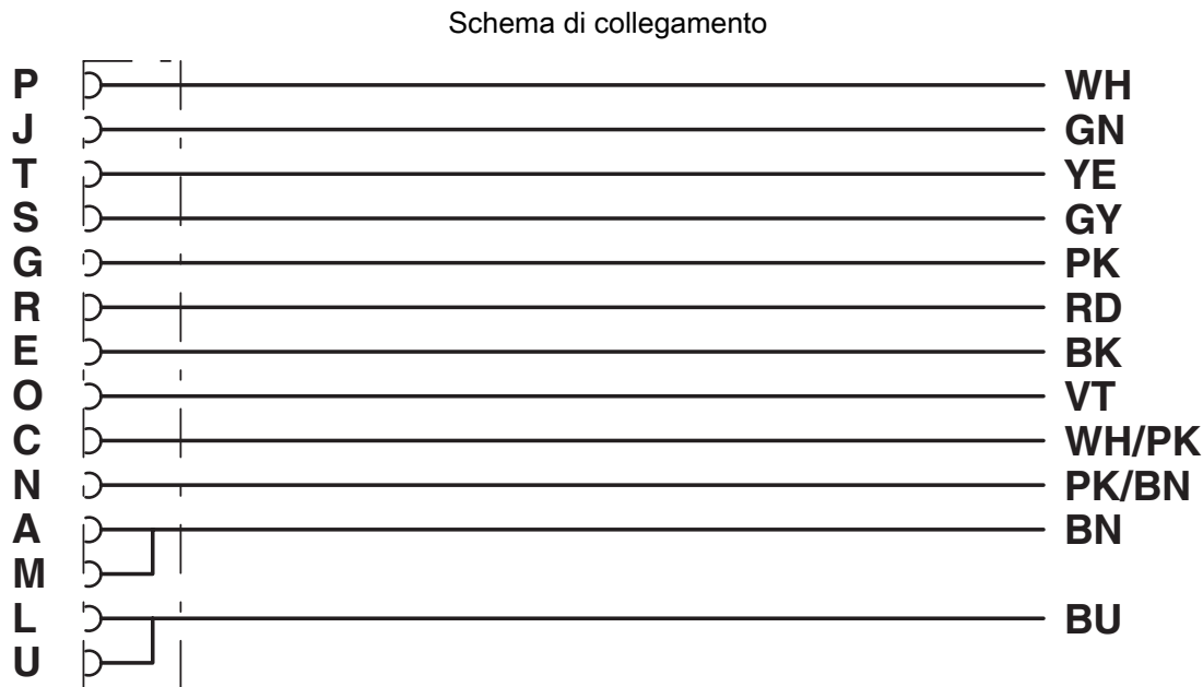
Equipaggiamento dei contatti del connettore femmina M16
