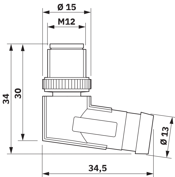
Disegno quotato
