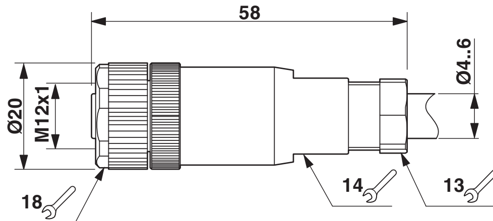
Disegno quotato
