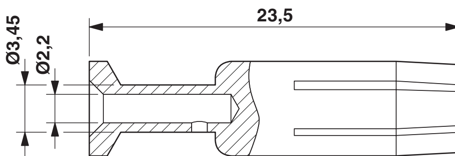
Disegno quotato
