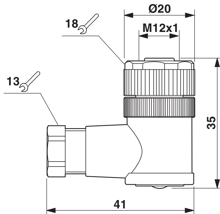
Disegno quotato
