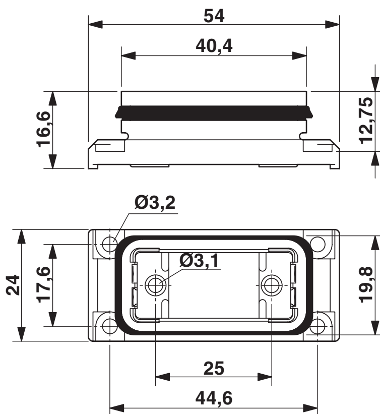
Disegno quotato
