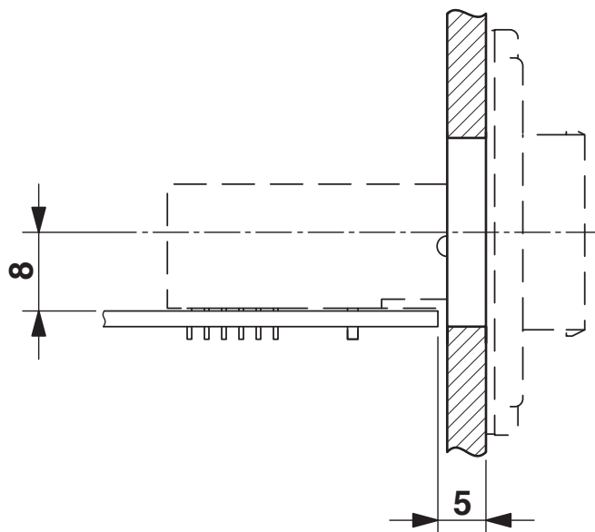
Disegno quotato
