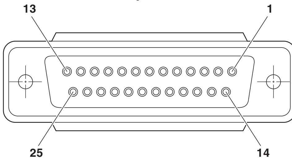
Disegno schema
