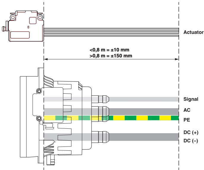
Disegno quotato
