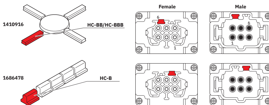
Disegno schema
