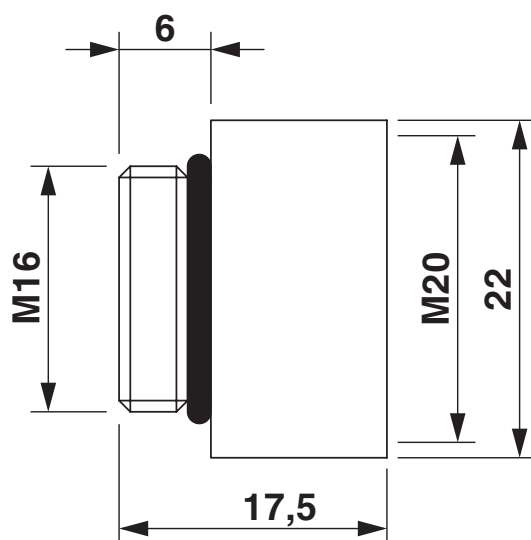
Disegno quotato
