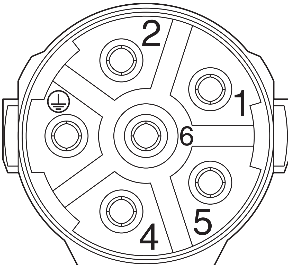
Disegno schema
