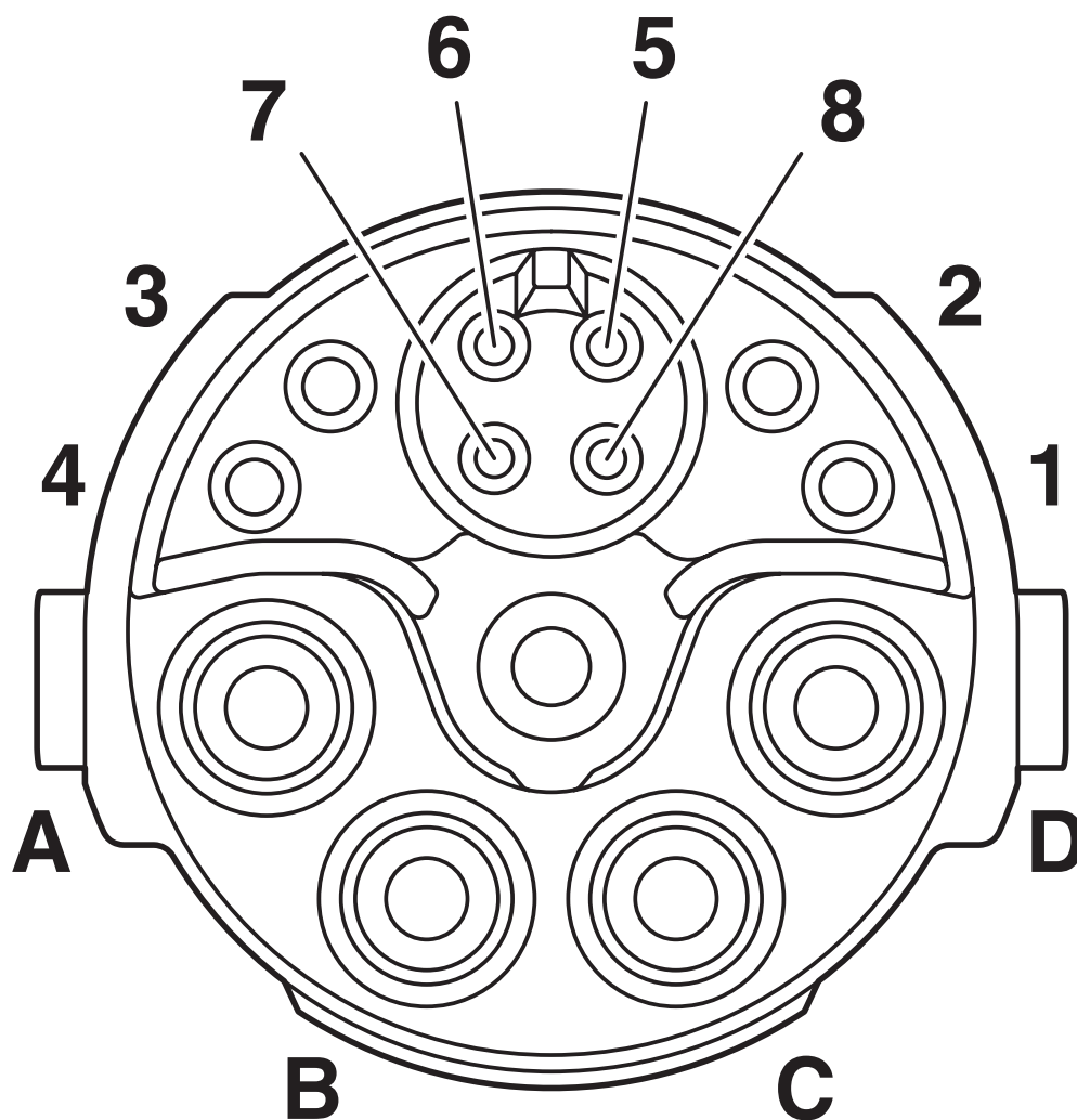
Pinning connettore femmina segnale
