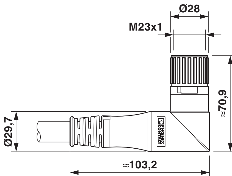
Disegno quotato
