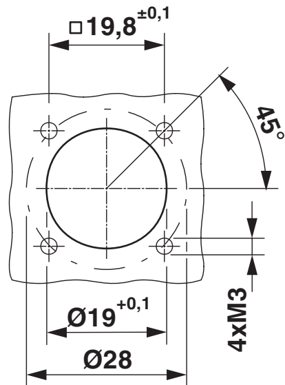
Disegno quotato
