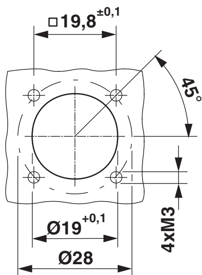
Disegno quotato
