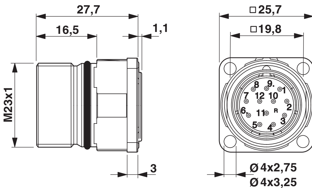
Disegno quotato
