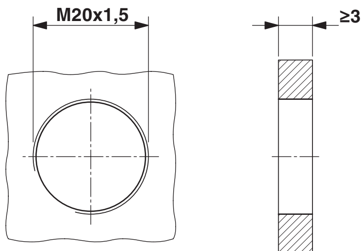
Disegno quotato
