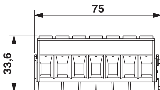
Disegno quotato
