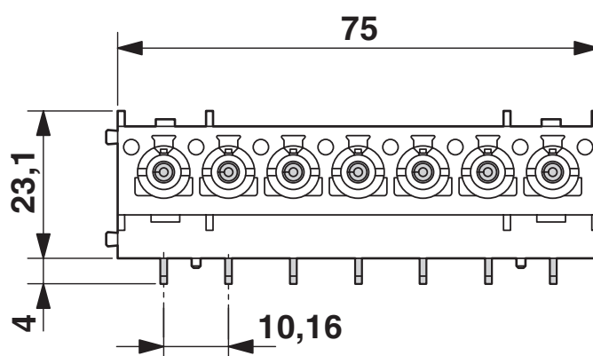
Disegno quotato
