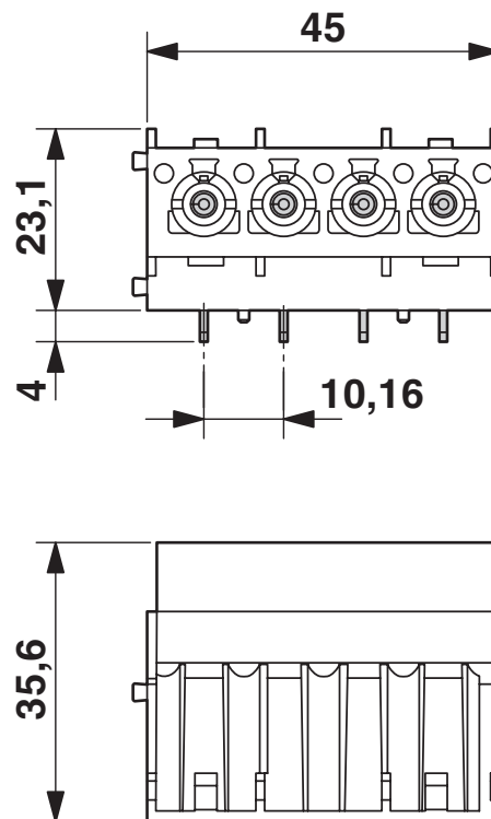
Disegno quotato
