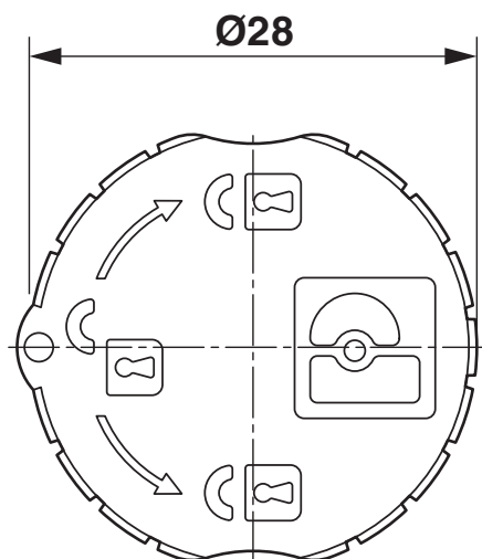
Disegno quotato
