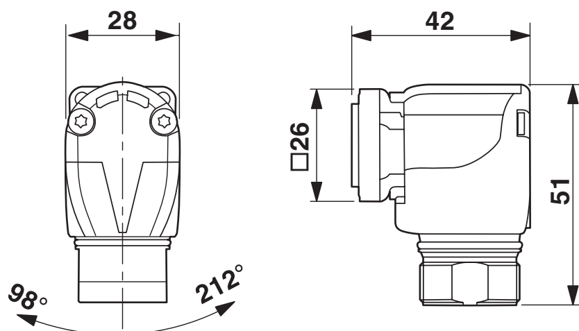
Disegno quotato
