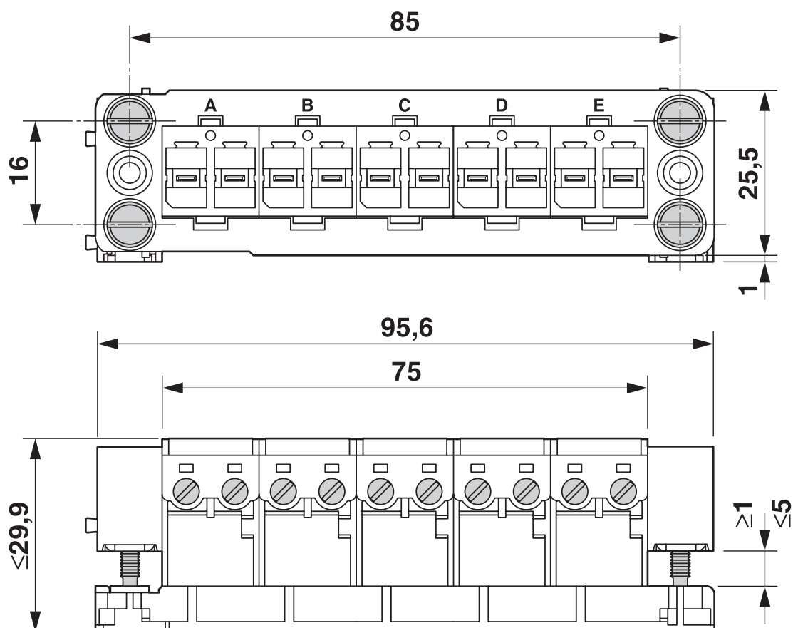
Disegno quotato
