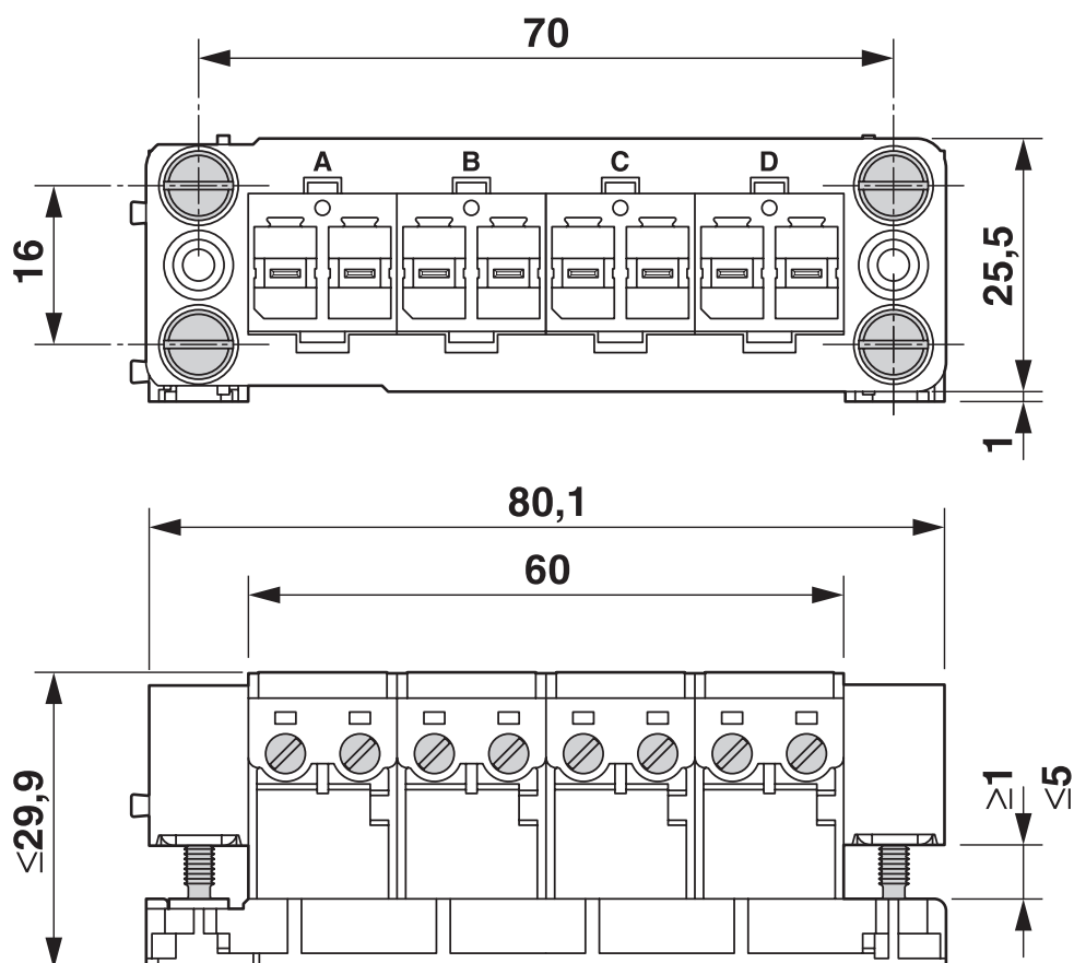
Disegno quotato
