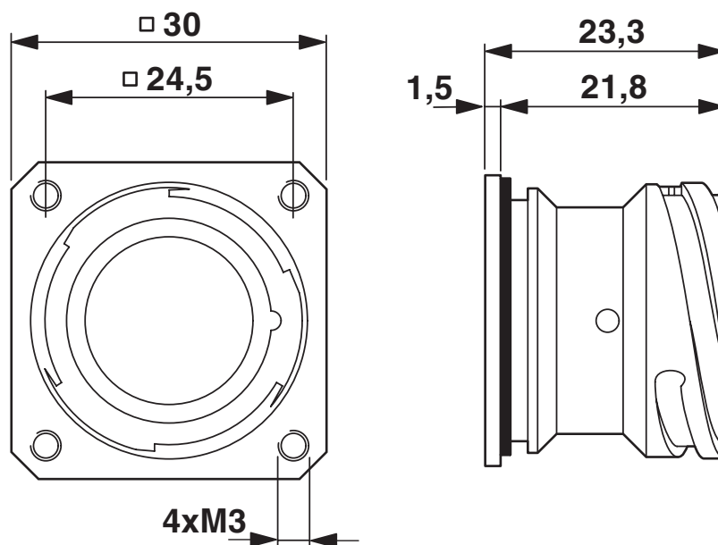
Disegno quotato
