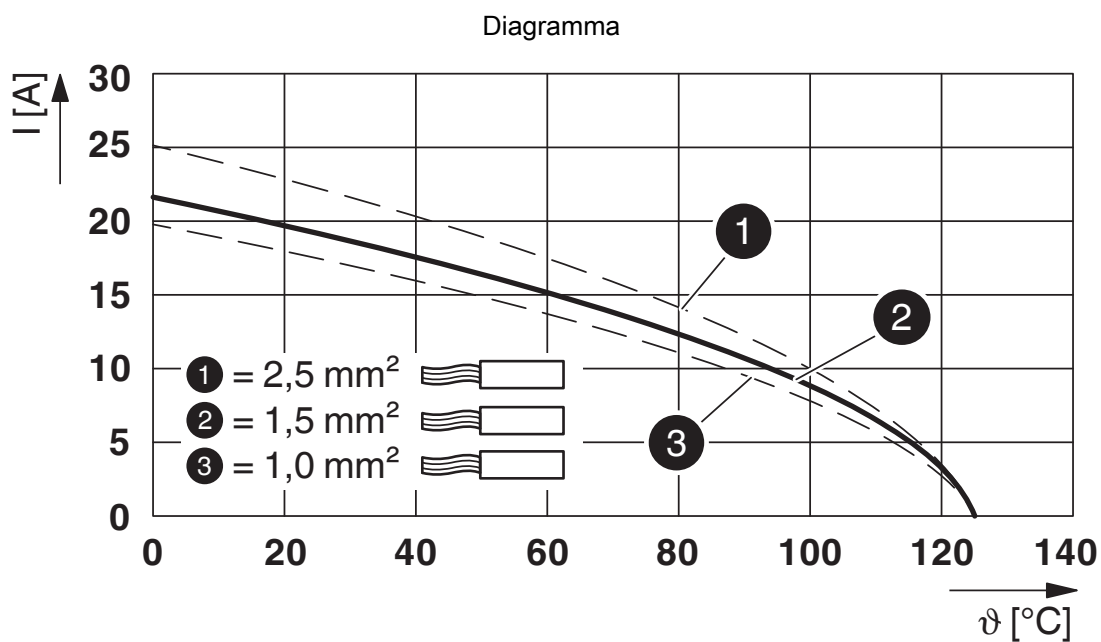
Diagramma di declassamento per conduttori rigidi
