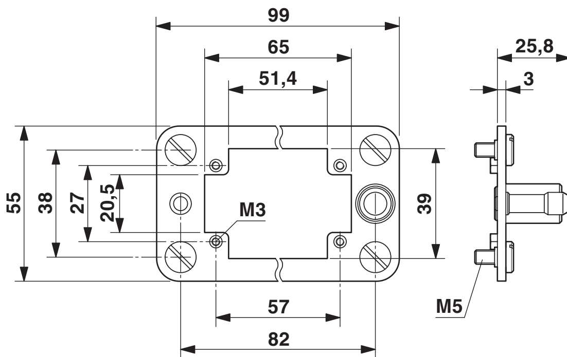
Disegno quotato
