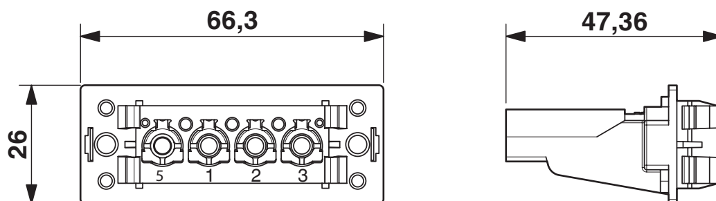
Disegno quotato
