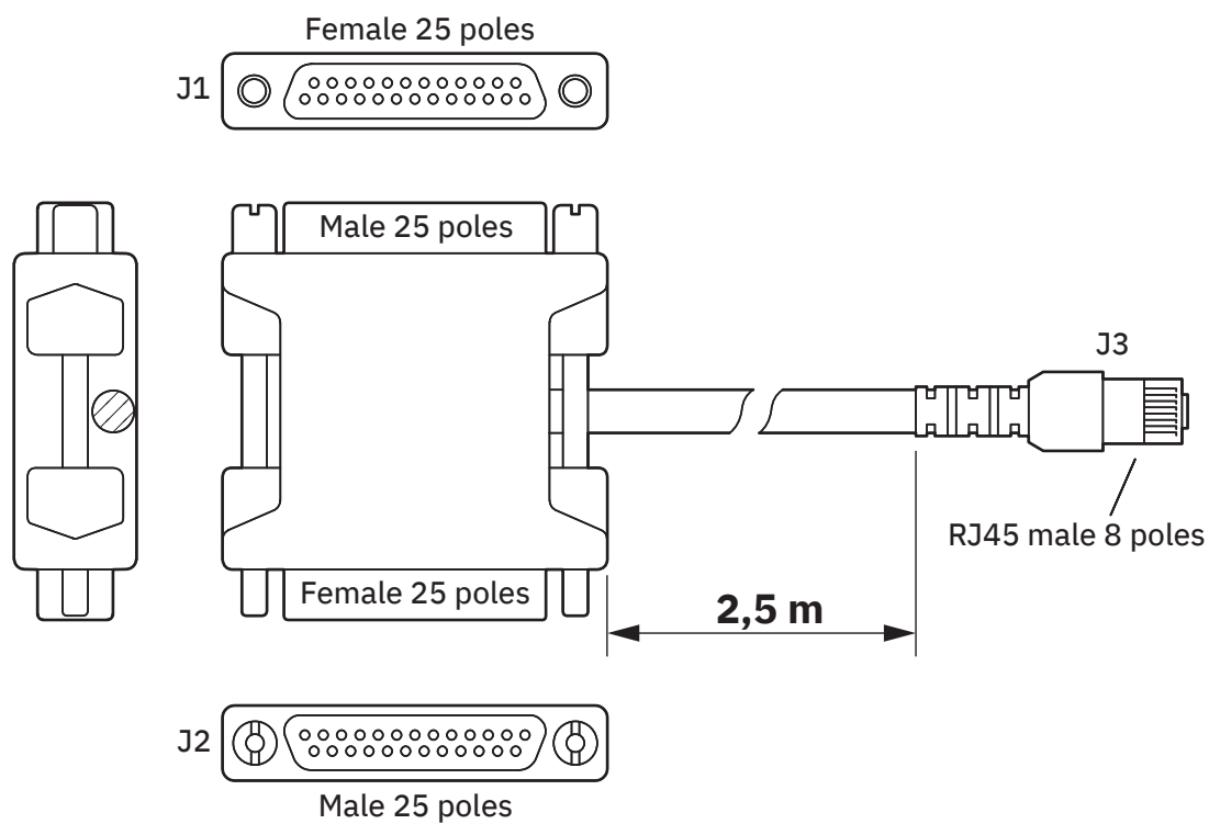
Disegno schema
