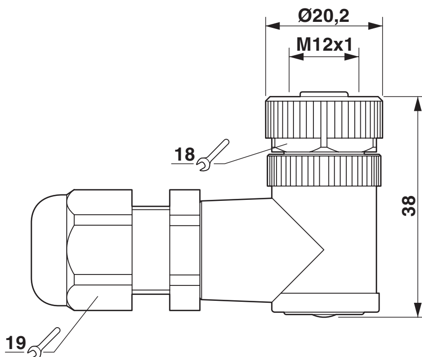
Disegno quotato
