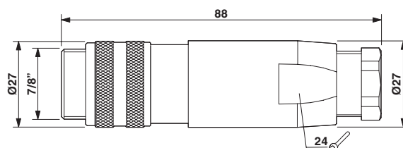
Disegno quotato
