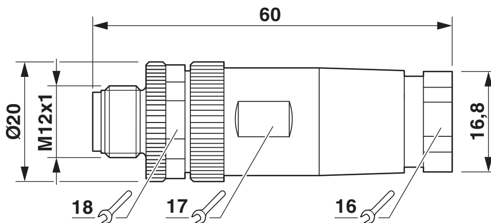
Disegno quotato
