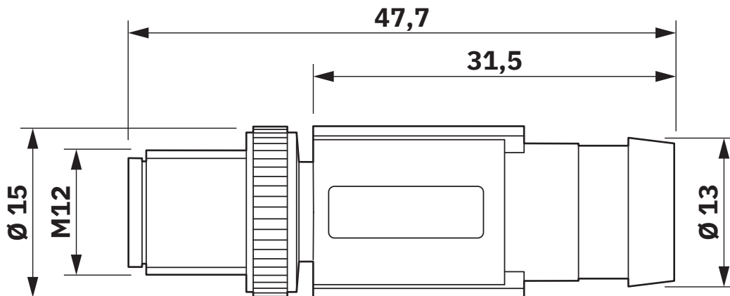
Disegno quotato
