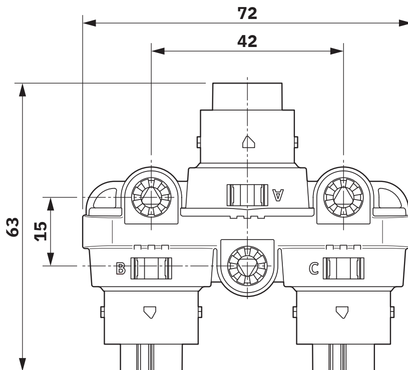
Disegno quotato
