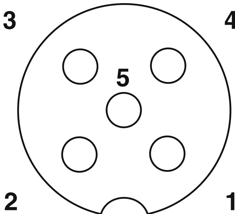
Assegnazione poli connettore femmina M12, a 5 poli, codifica A, visualizzazione lato femmina
