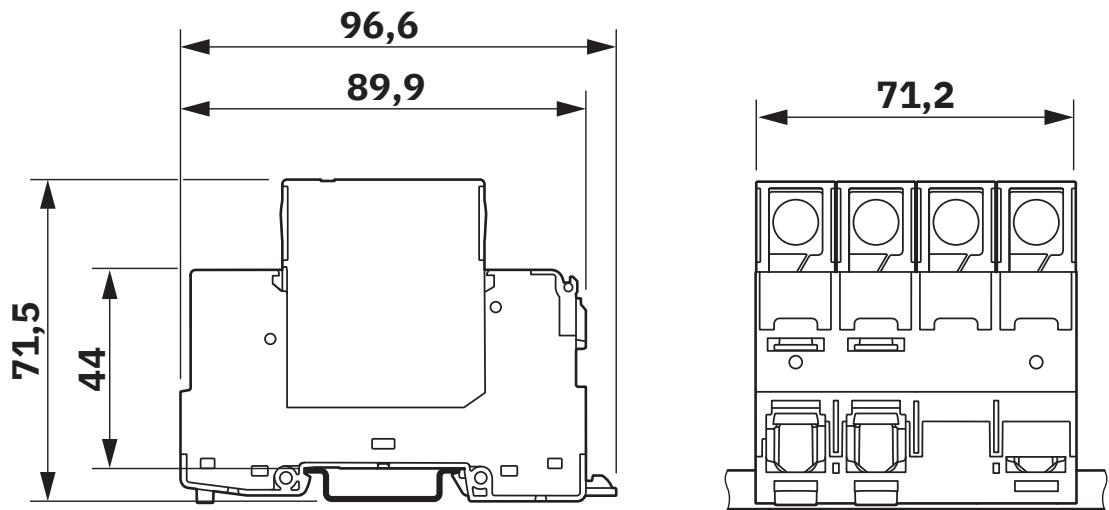
Disegno quotato
